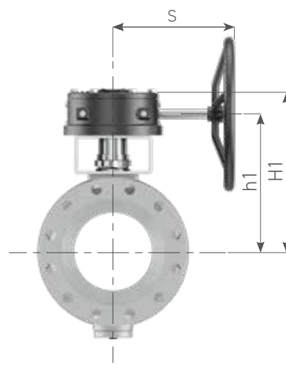
DN 250 Actuator - valve coupling / Accoppiamento valvola - attuttore ISO 5211
