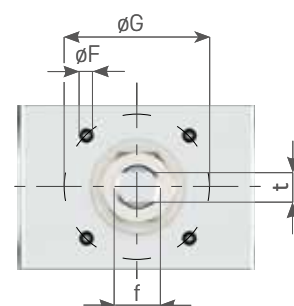
DN 200 Actuator - valve coupling / Accoppiamento valvola - attuttore ISO 5211
