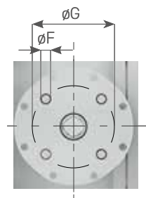
DN 250 Actuator - valve coupling / Accoppiamento valvola - attuttore ISO 5211
