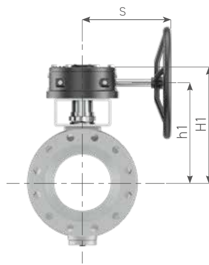
DN 250 - 300 Actuator - valve coupling / Accoppiamento valvola - attuatore ISO 5211
